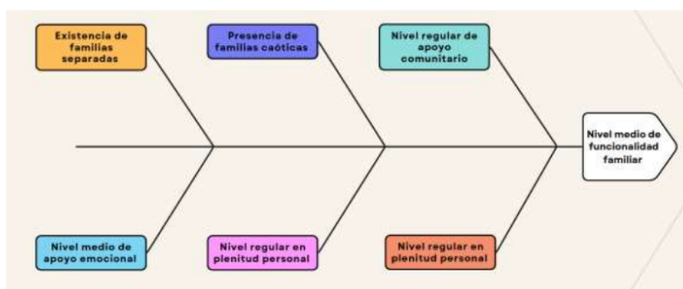
Figura 17 Diagrama Ishikawa
