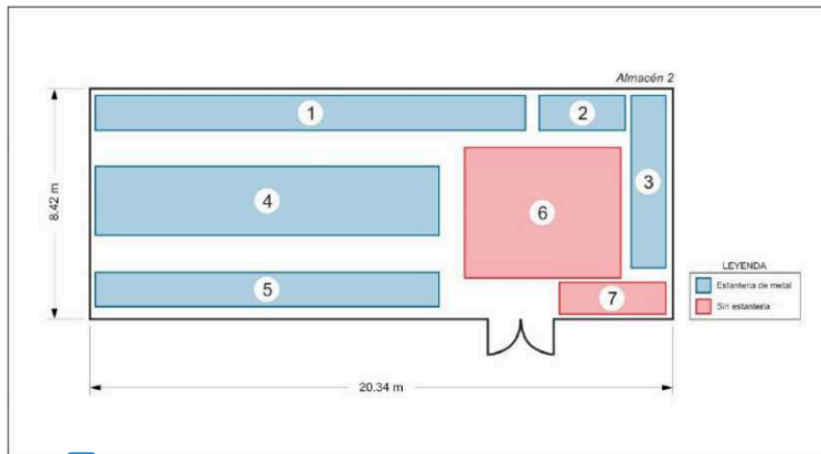
Figura 13 Distribución del almacén 2
