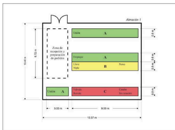
Figura 43 Layout propuesto del almacén 1
