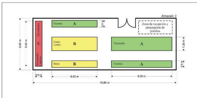
Figura 45 Layout propuesto del almacén 3
