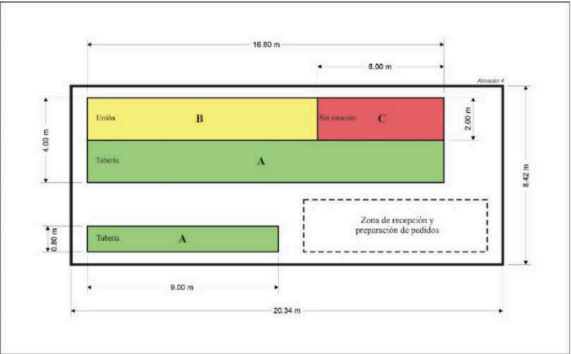
Figura 46 Layout propuesto del almacén 4
