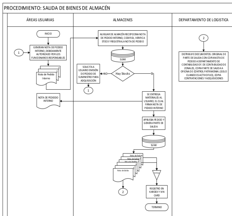
Figura 7 Flujograma de salida de bienes del almacén
