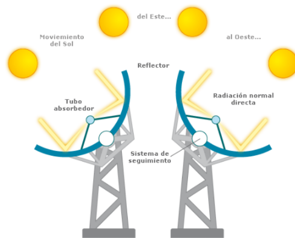
Figura 2.3. Reflector con sistema de seguimiento
