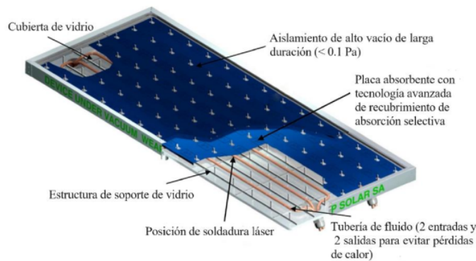
Figura 1.3. Esquema de colector de tubos evacuados
