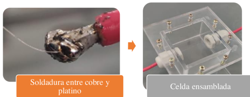
Figura 3.4. Conexiones eléctricas
