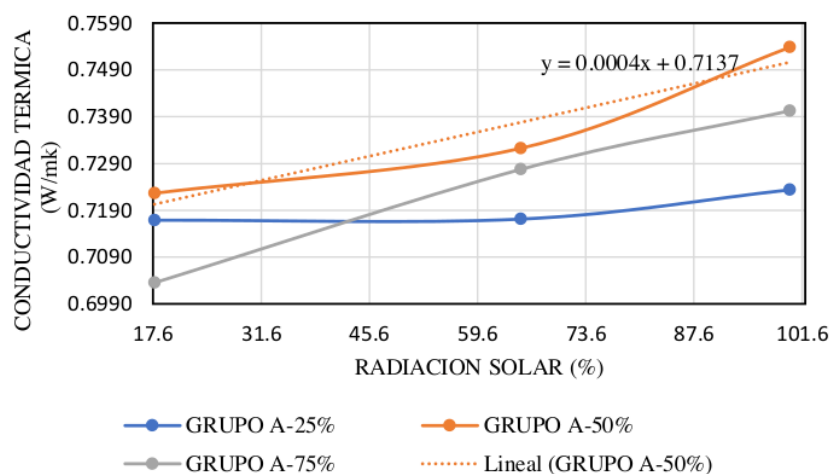
Figura 4. 17. Conductividad térmica Vs radiación solar del GRUPO A
