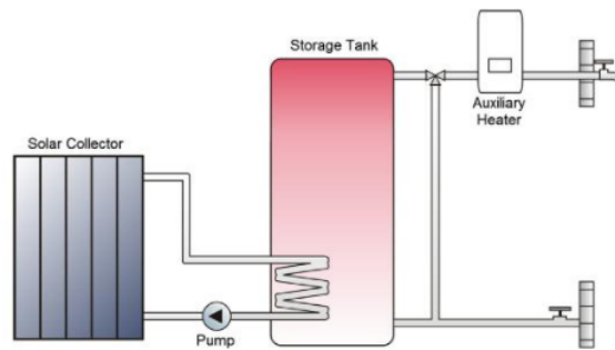
Figura 2.2. Esquema sistema solar térmico.
