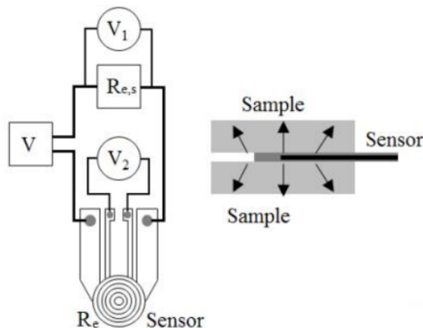
Figura 2. 6. Método de la fuente de plano transitorio
