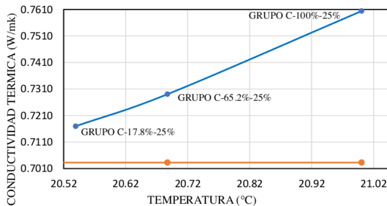
Figura 4.9. Conductividad térmica de la muestra GRUPO C-25%
