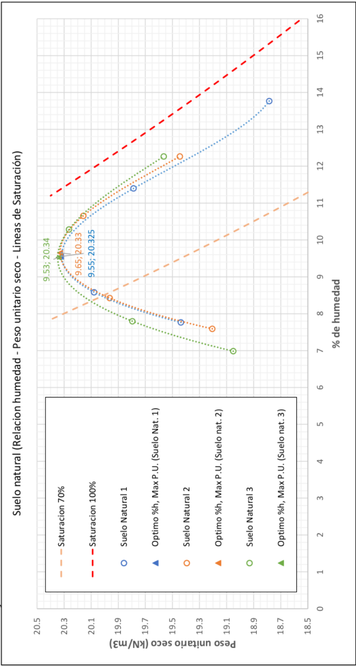
Figura 26 Ensayo de Proctor Modificado del suelo natural
