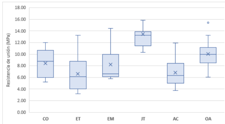
FIGURA N° 1: RESISTENCIA DE UNIÓN MICROTENSIL (MPa) EN FUNCIÓN DE LAS ESTRATEGIAS DE LIMPIEZA
