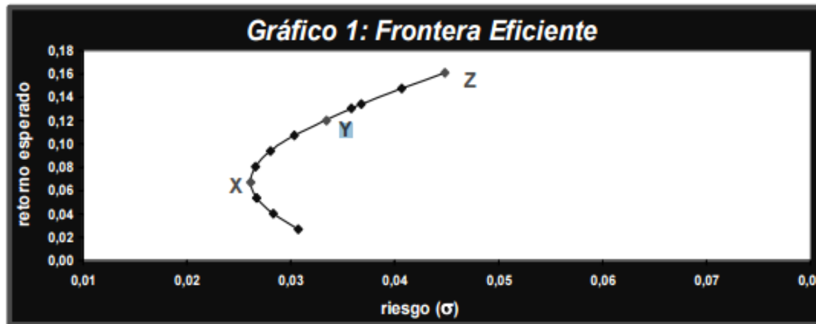
GRAFICO N°2 FRONTERA EFICIENTE
