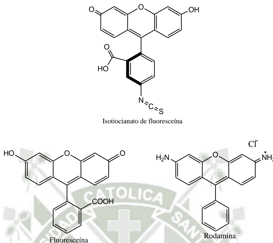
Fig. 4. Estructura de algunos colorantes orgánicos 31 .
