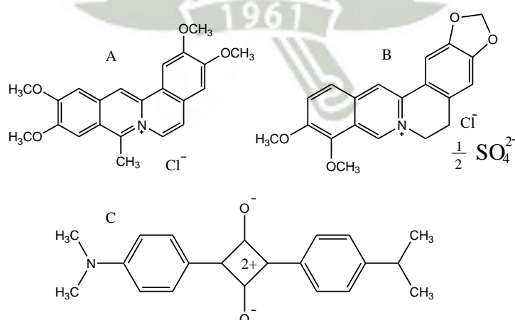
Fig.3. Estructura de fluoróforos 30 . A) coralina B) berberina C) squarylium.
