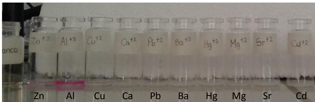
Fig. 29. Fenómeno colorimétrico que evidencia afinidad por Al^{3+} .
