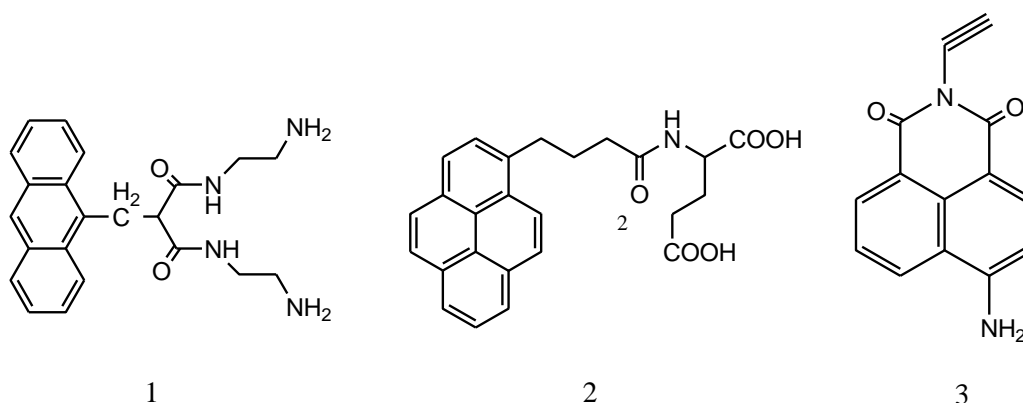
Fig. 2. Estructura de algunos quimiosensores fluorescentes para iones metálicos 29 .
