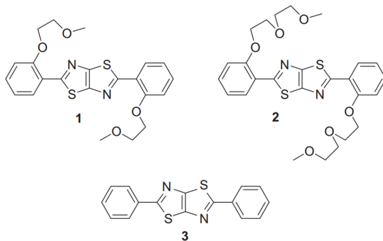
Fig. 8. Estructuras de derivados de tiazol 35 .
