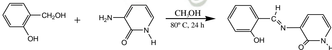
Fig. 6. Síntesis del quimiosensor 36 \text{C}_{12}\text{H}_{11}\text{O}_2\text{N}_2 (HL).
